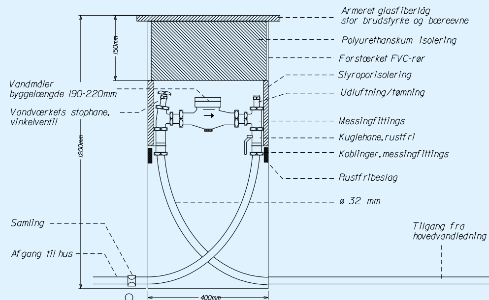
Snit af målebrønd 1:10
