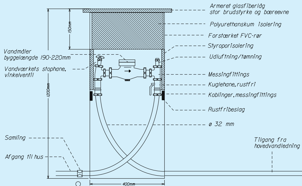
Snit af målerbrønd 1:10
